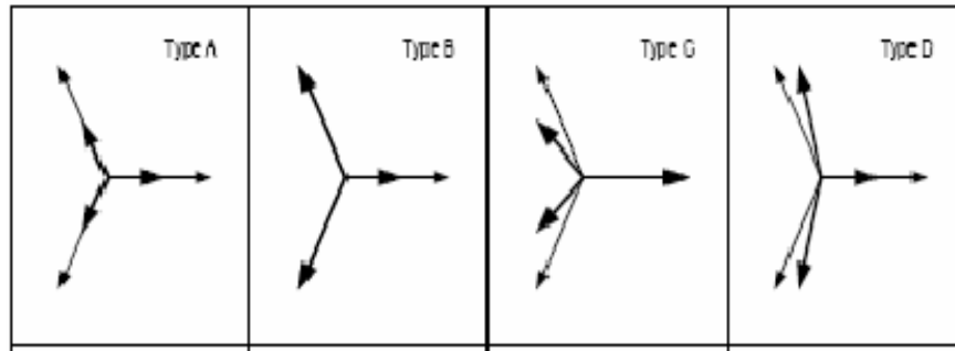
Fig. 2 Different types of sags: (a) type A (b) type B (c) type C (d) type D
